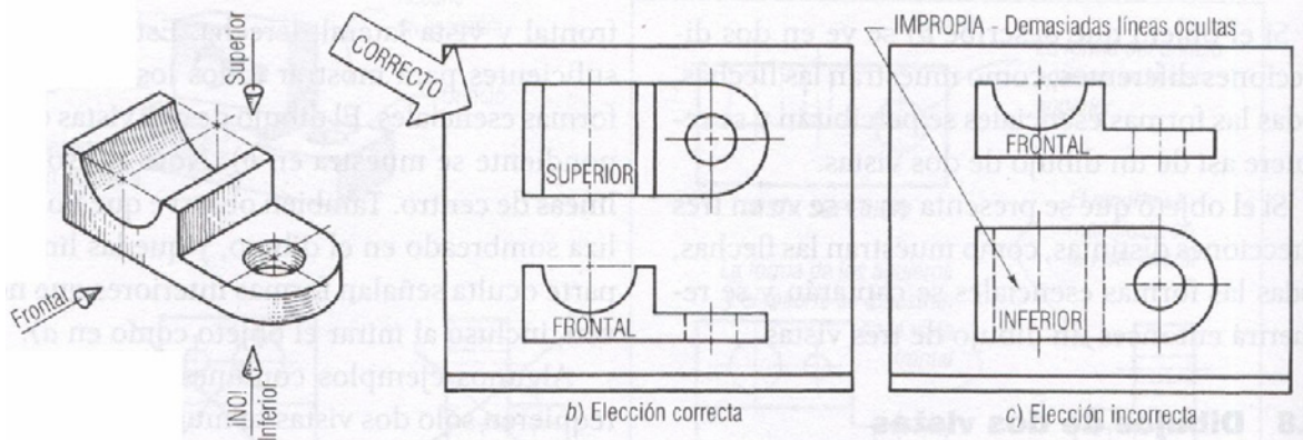
Vistas con el menor número de líneas no visibles.
