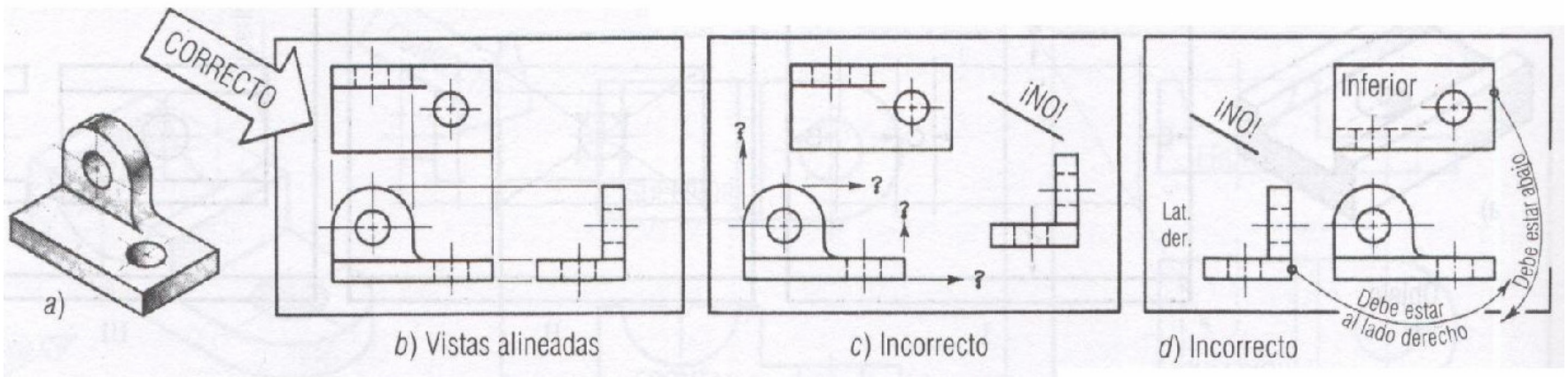
Disposición de las vistas.
